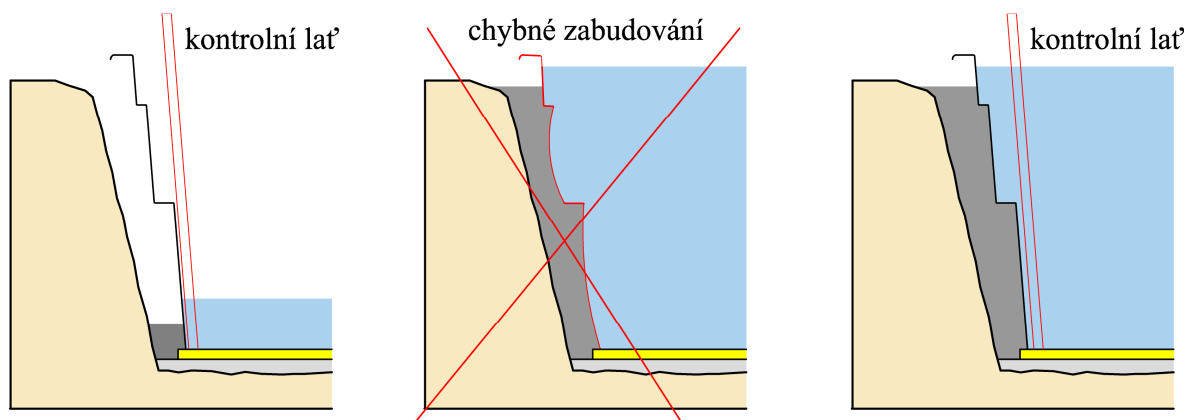
kontrola rovinnosti stěn ve svislém směru
