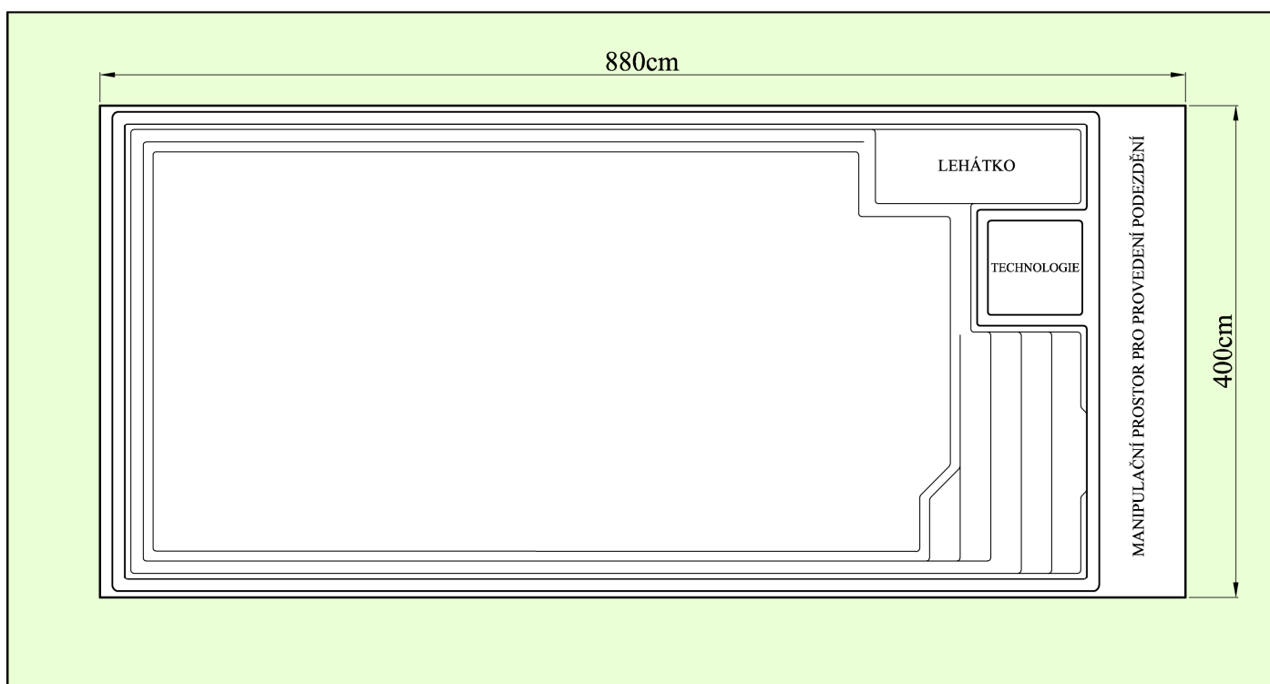
půdorys výkopu
