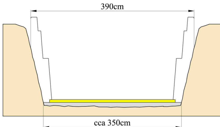
příčný řez výkopem - šířka betonové desky cca 350cm
